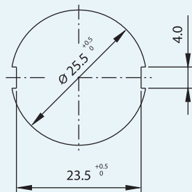
(Ø25)
